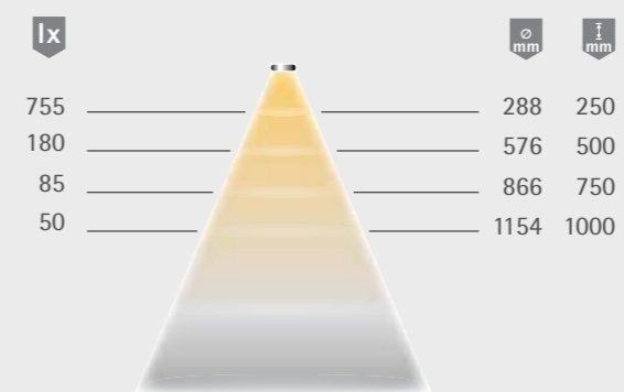
Lichtverteilungsdiagramm 60°
